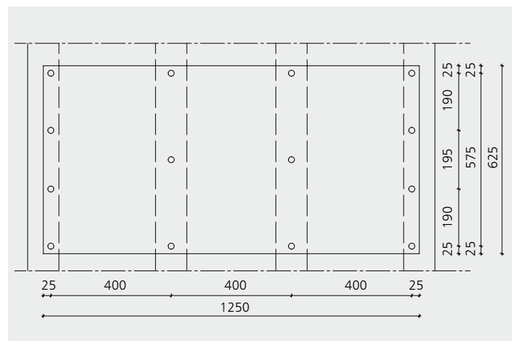
Schraubbefestigung
